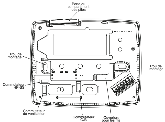
Figure 1. Socle du thermostat
