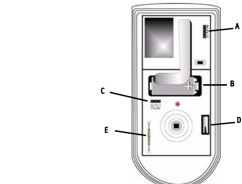
Fig. 2 Componenti del sensore di movimento passivo ad infrarossi ES1260
