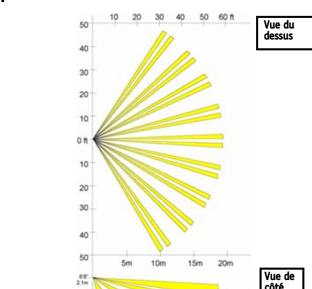
Fig. 3 Carte des zones du ES1260 </
