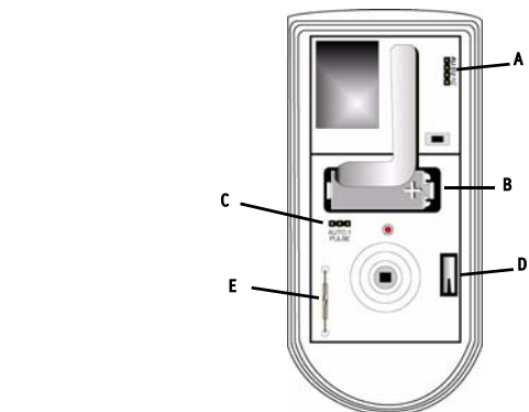
Fig. 2 ES1260 Komponenter
