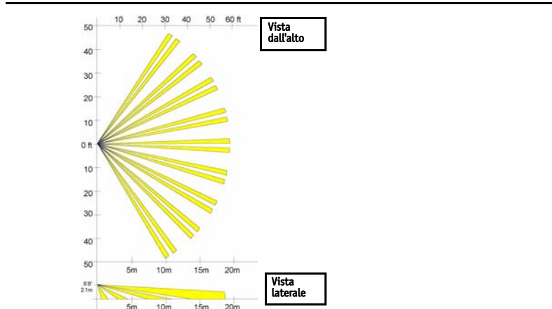
Fig. 3 Mappa zone dell'ES1260
