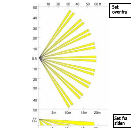
Fig. 3 ES1260 Dækningsmønstre
