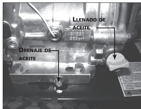
Figura 15 - Puntos de drenaje y llenado
