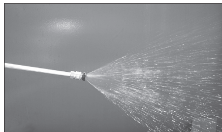
Figura 13 - Patrón de abanico ancho
