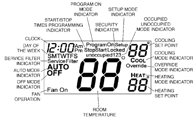
Fig. 1 — Thermostat Display
