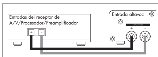
Figura 1 POLARIDAD
